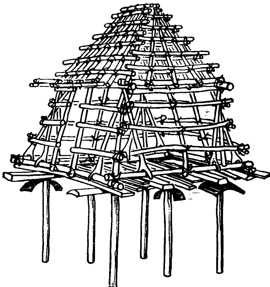
Конструкция амбара
